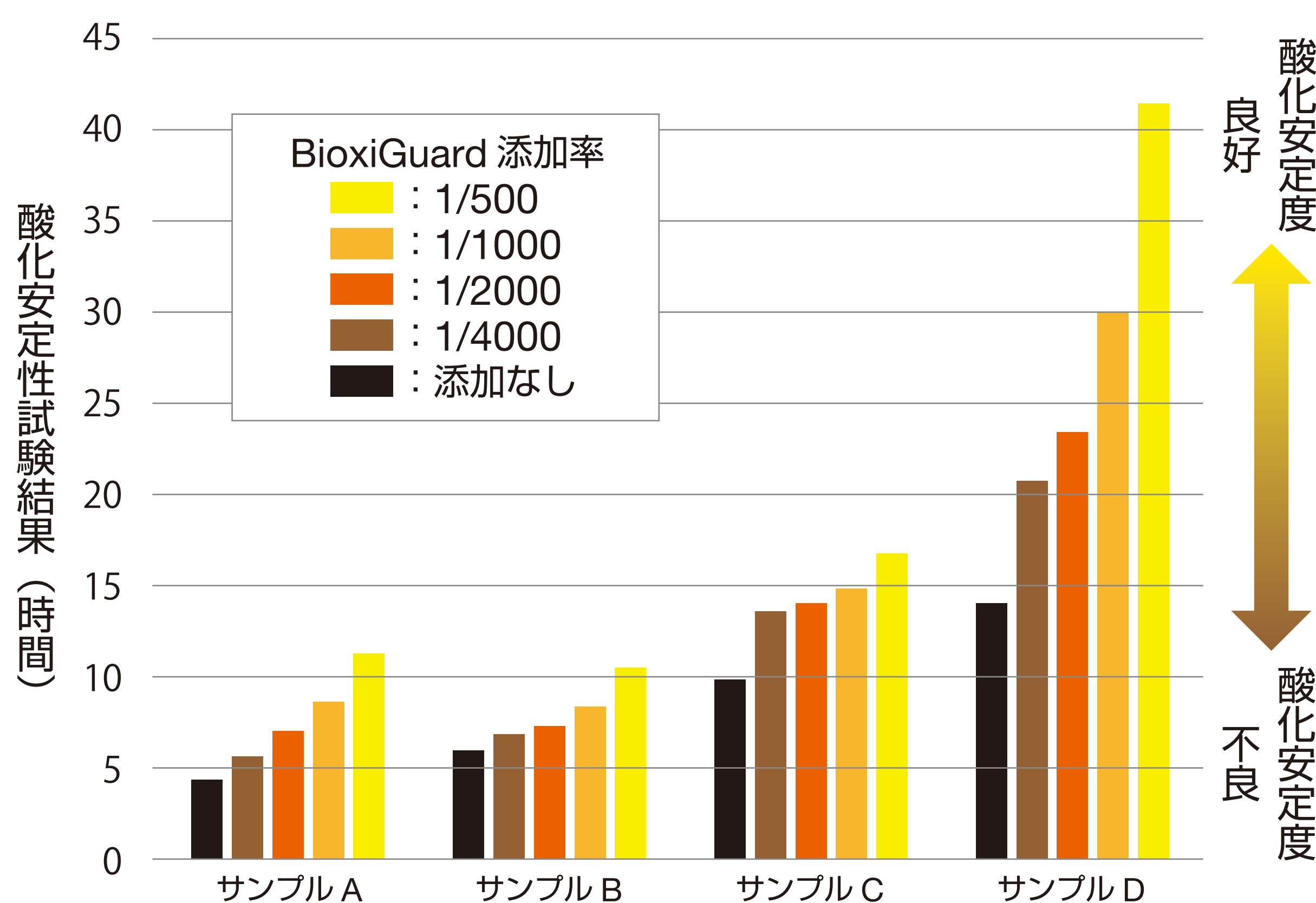
バイオディーゼル燃料に BioxiGuard を添加したときの 酸化安定性試験結果
