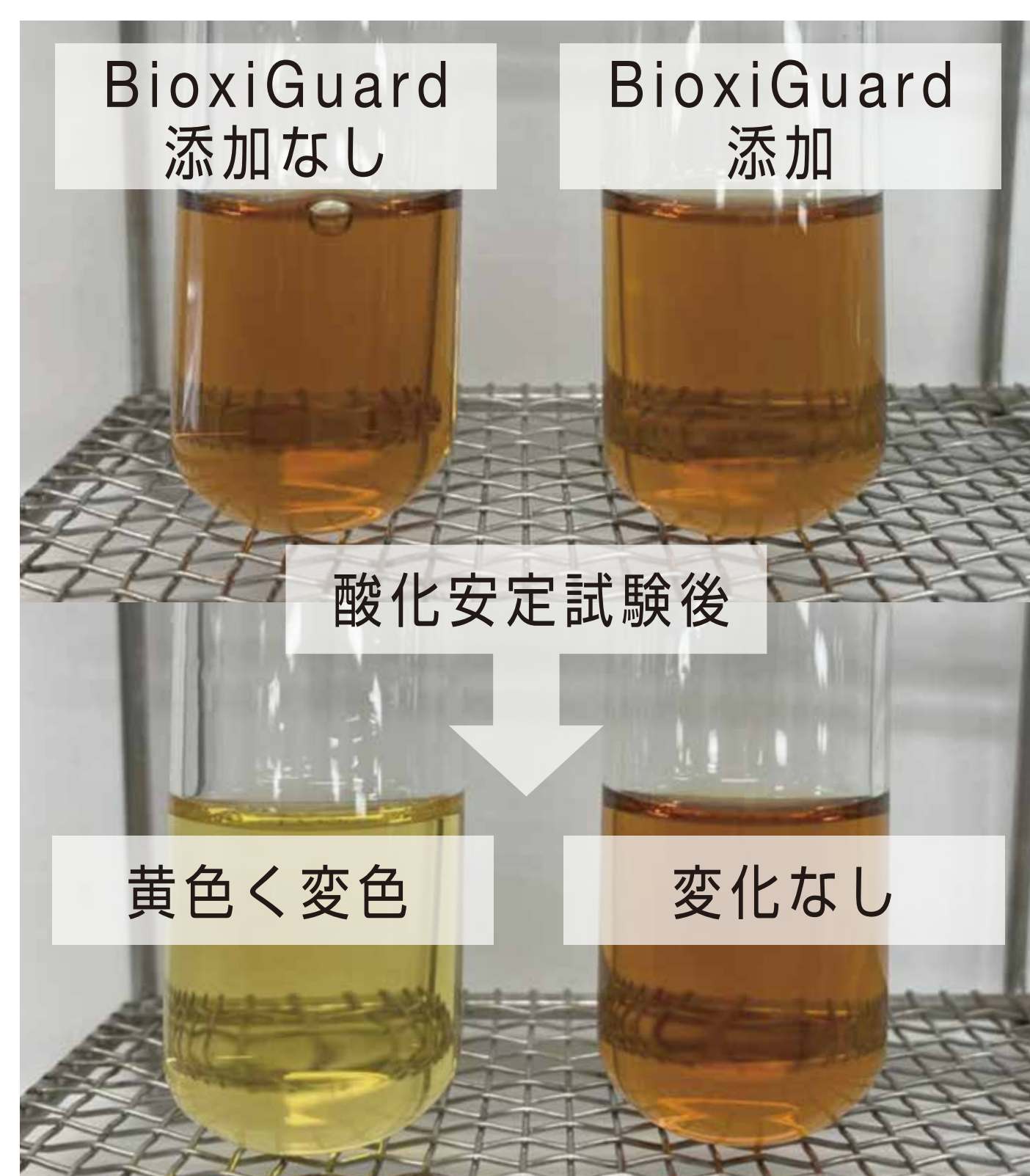
酸化安定性試験後のバイオディーゼル燃料 〈8時間・110℃で空気をバブリング(10L/h)〉
