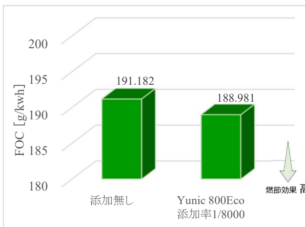
陸上の実験用船用2サイクル機関による燃焼試験結果 (燃費削減効果：最大 約1.2%)
