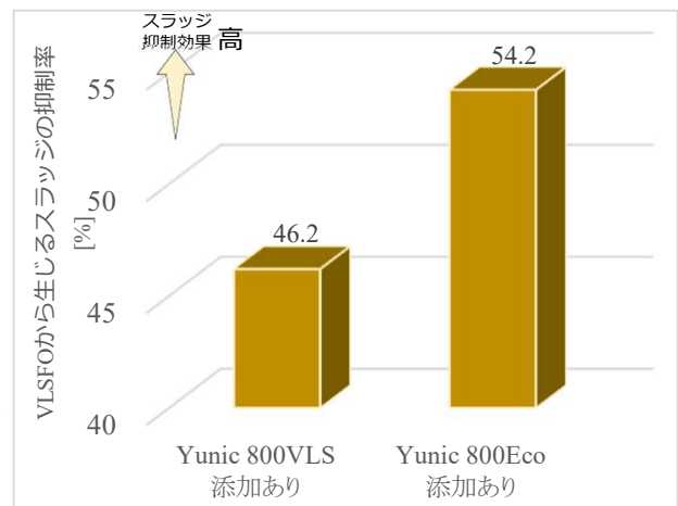
VLSFOを用いたスラッジ抑制効果 (50例以上の平均値) (スラッジ抑制効果は従来製品に比べ約20%改善)
